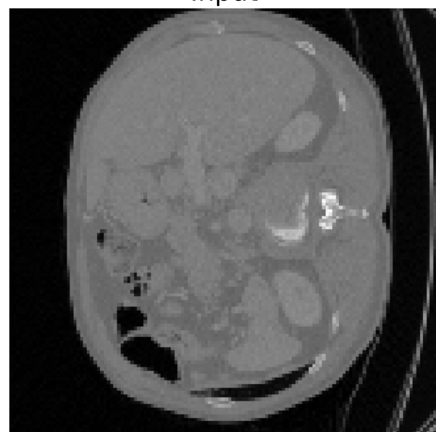
Input
